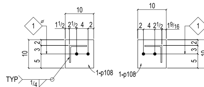
Section A-A 1015FR1
